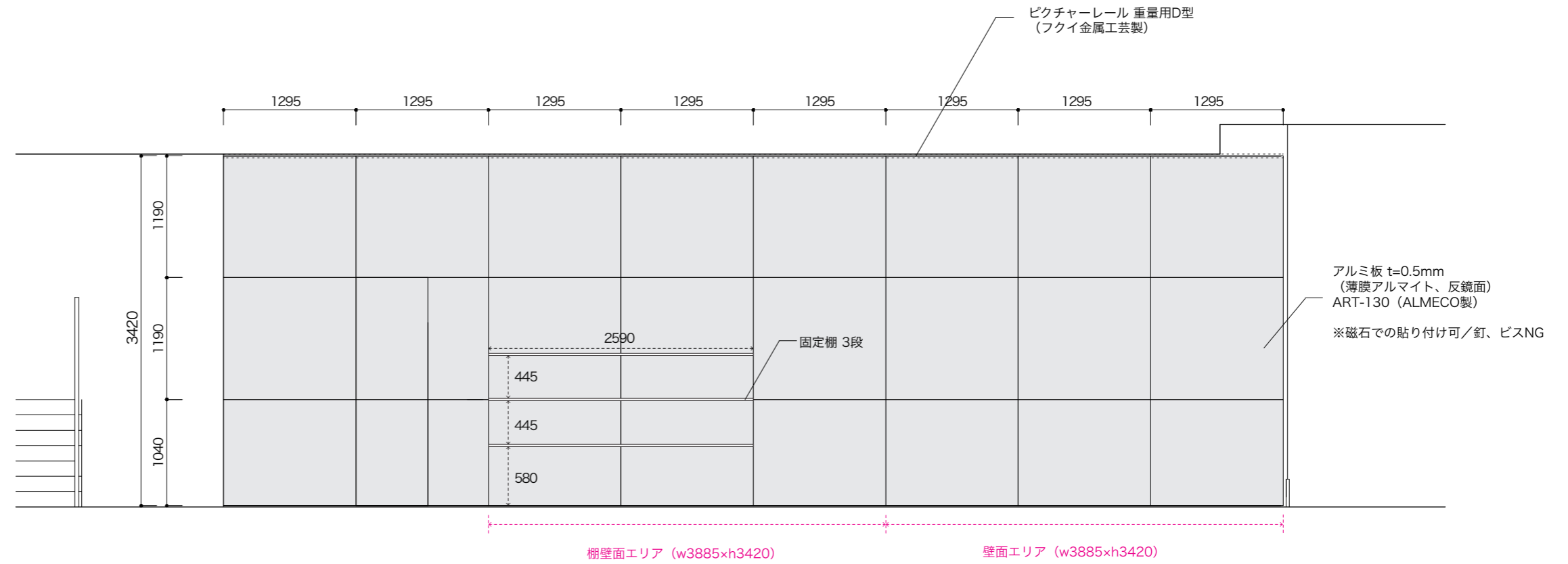
立面図 (1/50)
