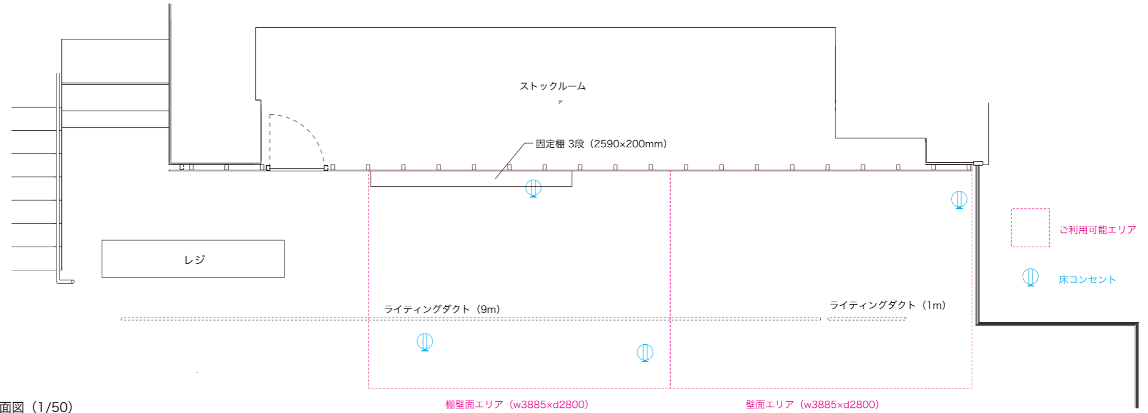
平面図 (1/50)
