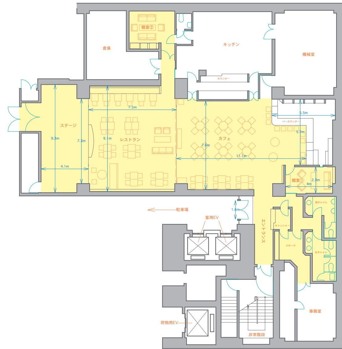
B1F レストラン CAY平面図
