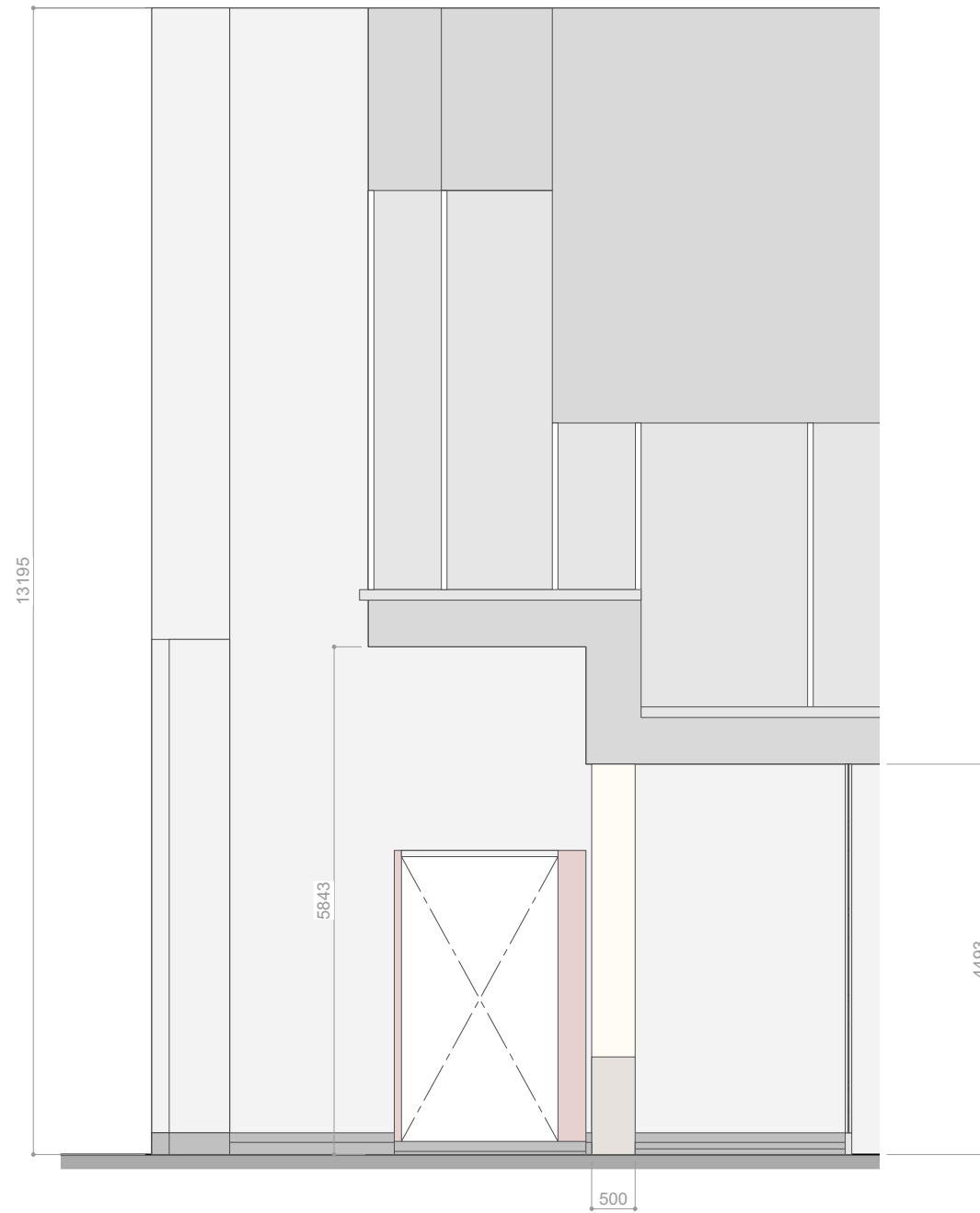
B elevation
