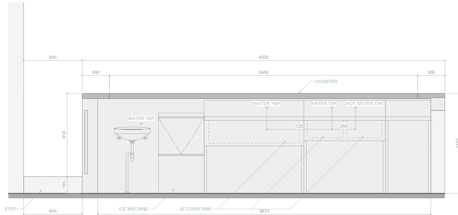
E elevation
